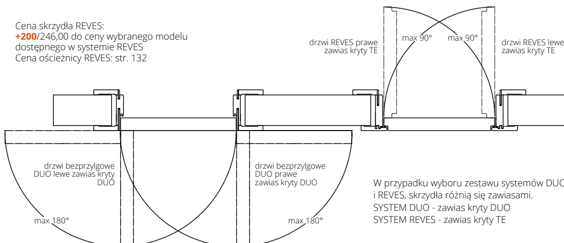
zawias kryty DUO, kolor srebrny - system DUO
